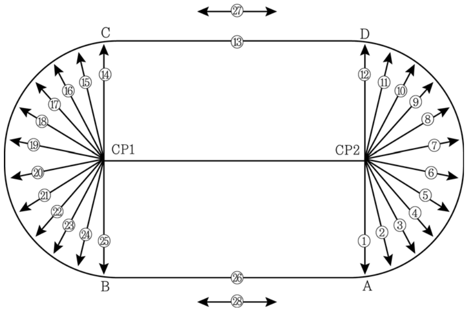
400m 표준트랙의 28포인트 컨트롤 계획
